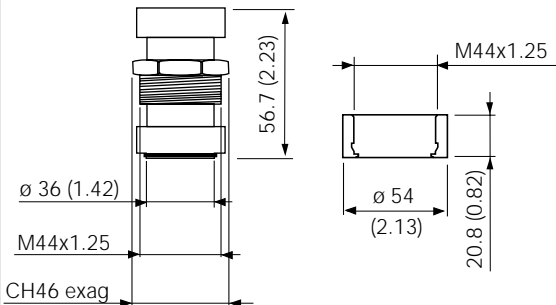
Fig. 40 - Threaded spud
