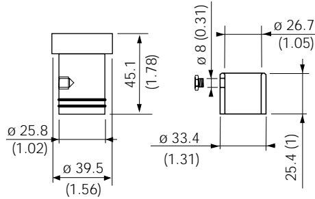
Fig. 38 - 1-screw spud
