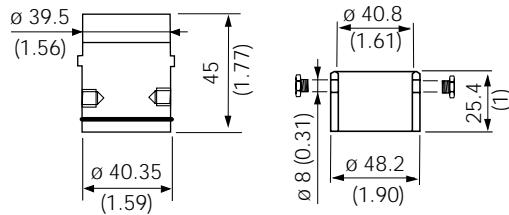
Fig. 39 - 2-screw spud
